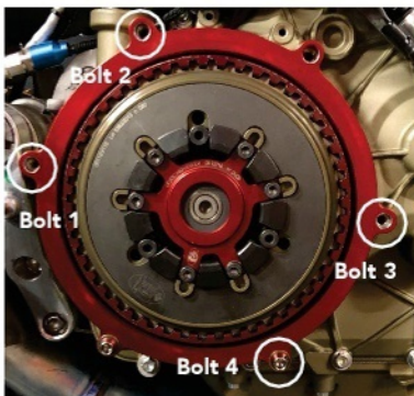
FIG 4. Trockenkupplung ohne Deckel
