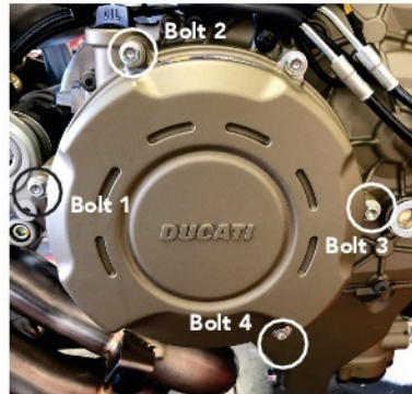
FIG 3. Sobald die Verkleidung entfernt wurde die 4 Schrauben entfernen und aufbewahren.
