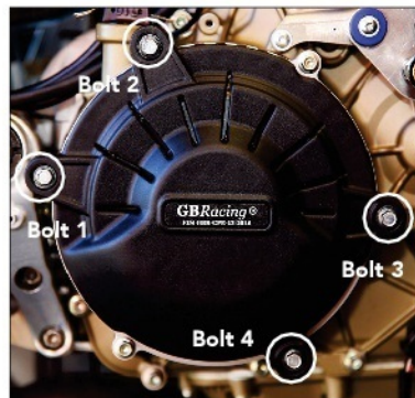
FIG 5. GBRacing cover über der Trockenkupplung montiert
